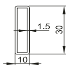
Waagerechte Rohren
