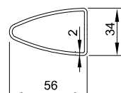
Vertikale Sammelrohren
