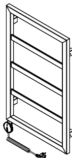
Boston EBO 555x904 konfiguracja lewa rys. aksonometryczny
