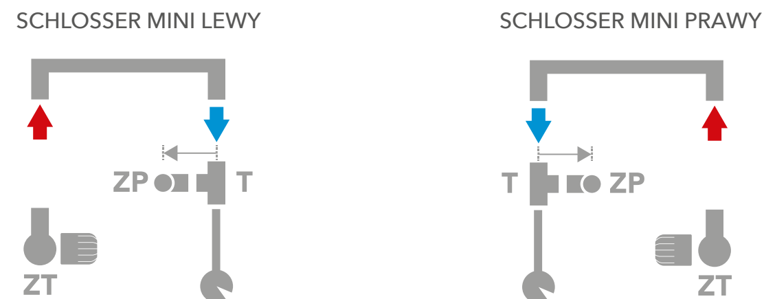
SCHEMAT IV SCHLOSSER MINI TERMOSTATYCZNY
